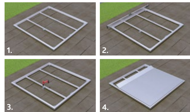
1. Montaža okvirja 2. Povezava nastavljivih nog in okvirja 3. Pritrditev nastavljivih nog v podzemlje 4. Pritrditev aluminijastih talnih plošč
